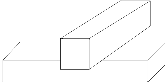
FIGURE 1. A non Lipschitzian domain
